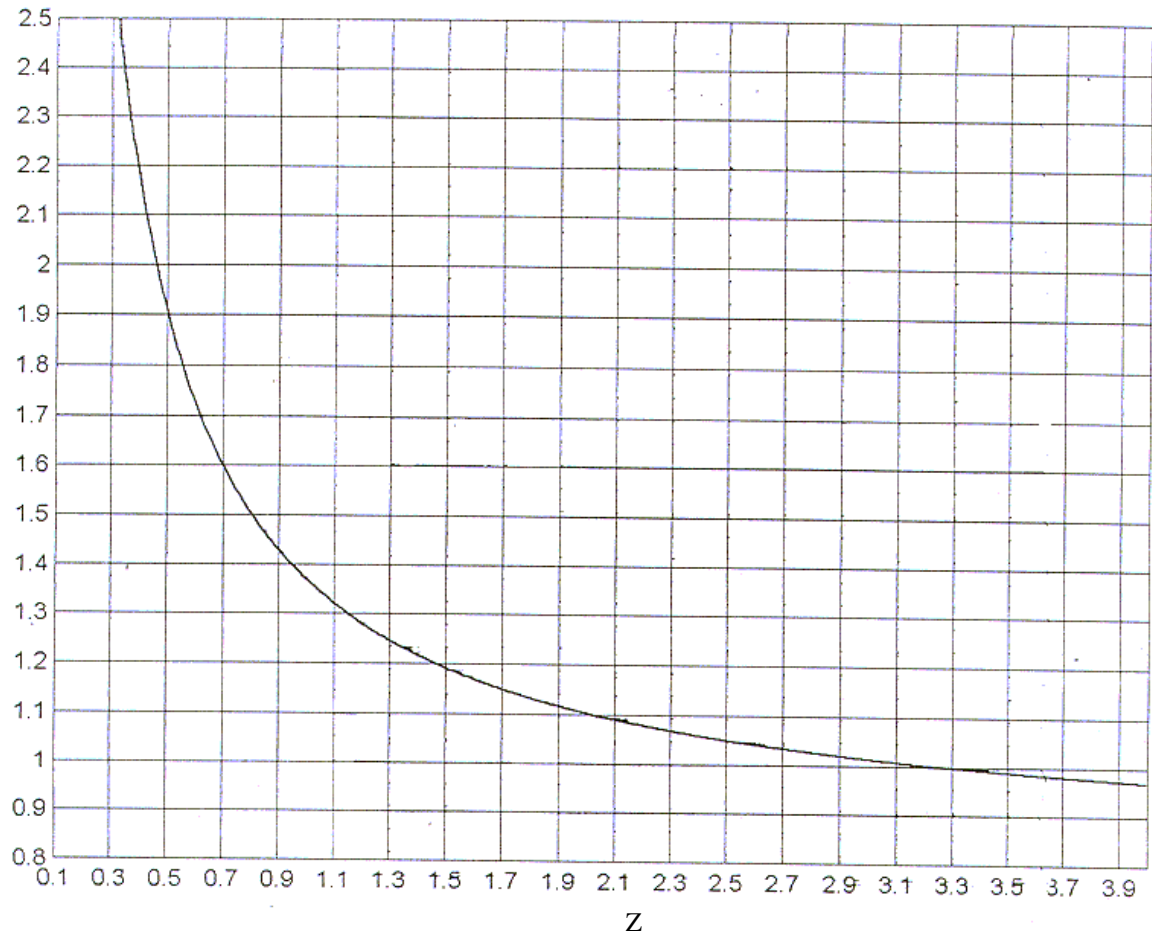
Рис.2.5. График для определения коэффициента C, используемого для вычисления весенней влажности.
