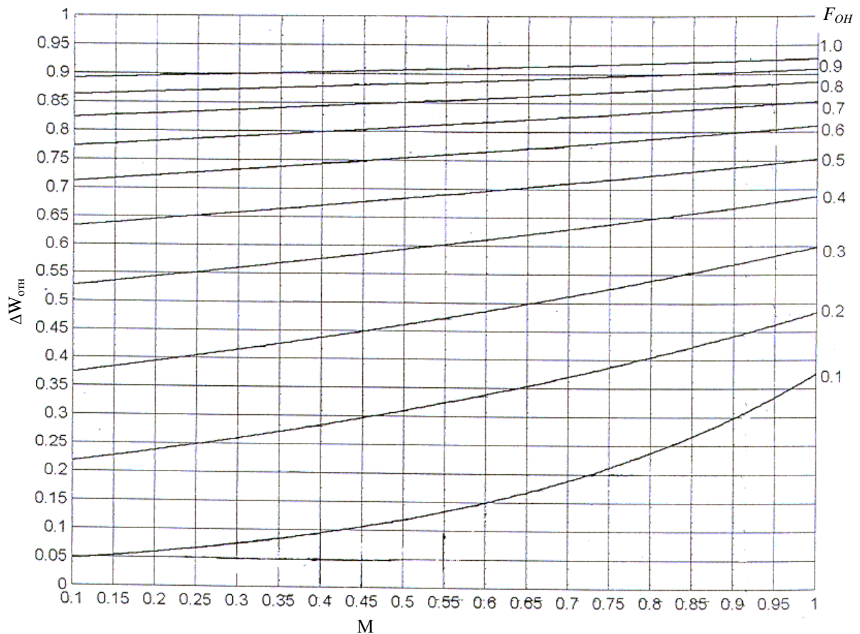
Рис.2.4. Номограмма для определения \Delta W_{отн} при значениях F_{он} и M .
