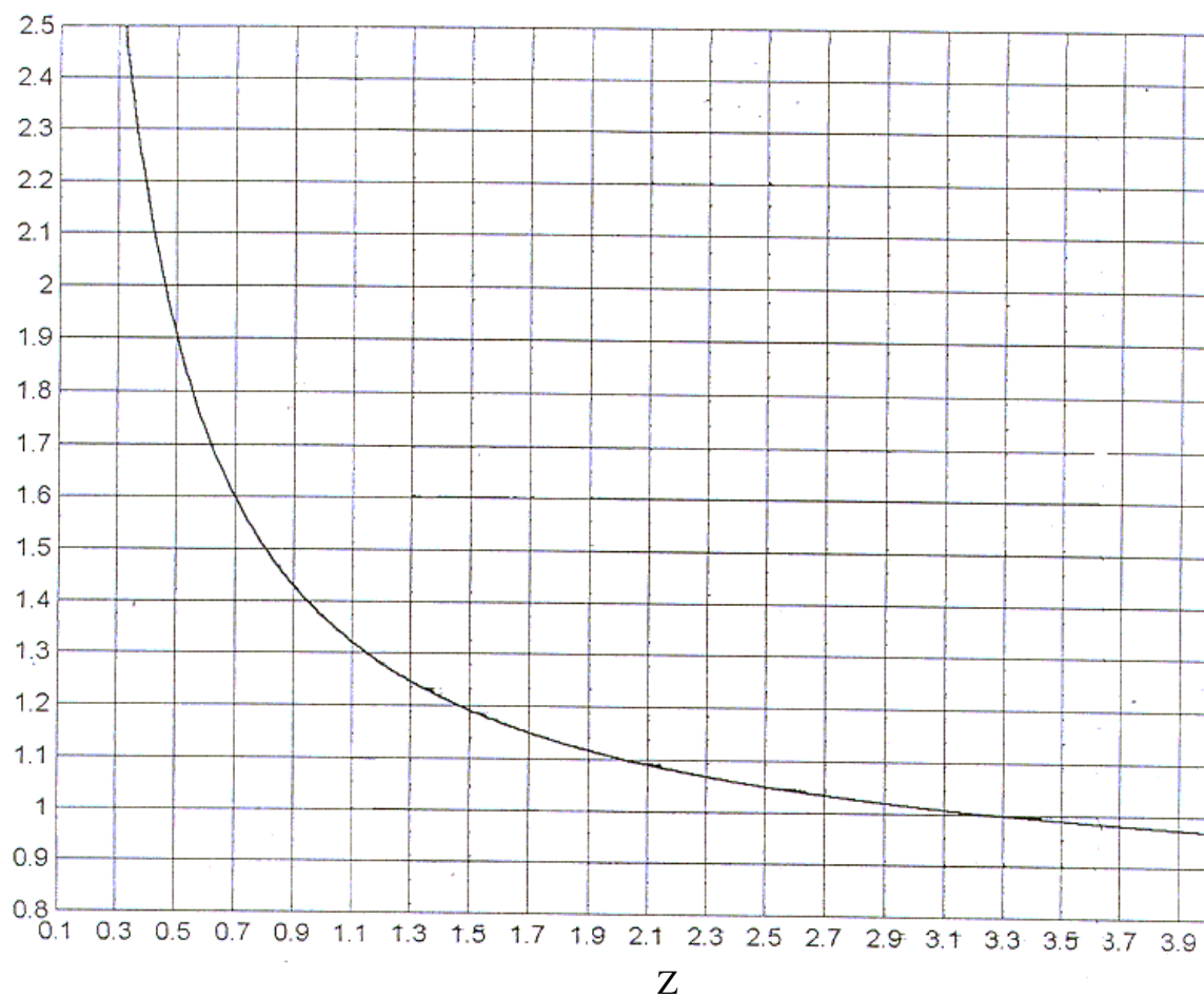
Рис.П.1.5. График для определения коэффициента С, используемого для вычисления весенней влажности.
