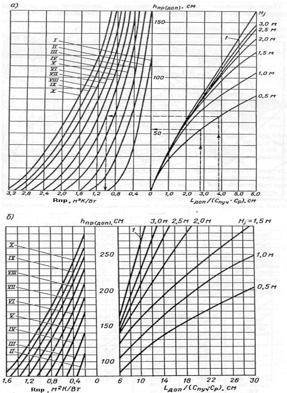
Рис.2.3. Номограмма для определения приведенного термического сопротивления дорожной одежды R_{пр} : I-X — номера изолиний на карте (рис.2.2); 1 — кривая расчета для 1-ого и 2-ого типов увлажнения рабочего слоя земляного полотна; H_j — глубина залегания расчетного УГВ от низа дорожной одежды, включая морозозащитный слой.
