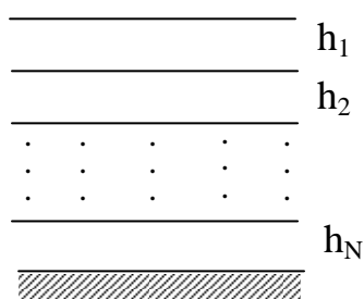
Рис.3.1. Расчетная схема для центральной части дорожной конструкции.
