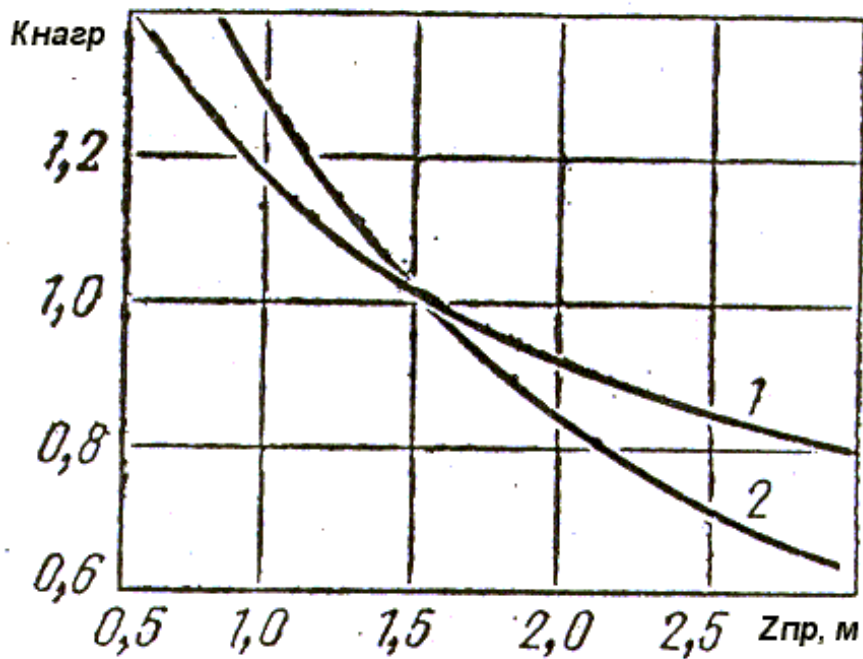
Рис.П.1.3.. Зависимость коэффициента K_{нагр} от глубины промерзания z_{гр} от поверхности покрытия. 1 – супесь тяжелая и пылеватая; суглинок; 2 – песок; супесь легкая, крупная
