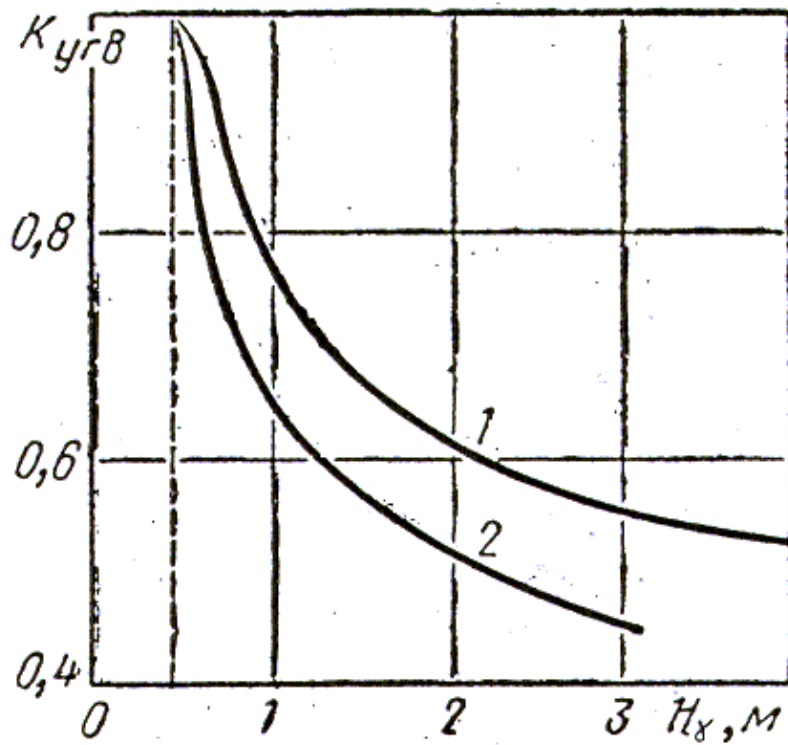
Рис.П.1.2. Зависимость коэффициента K_{угв} от расстояния от низа дорожной одежды до расчетного УГВ или УПВ. 1 – супесь тяжелая и тяжелая пылеватая, суглинок; 2 – песок, супесь легкая и легкая крупная.
