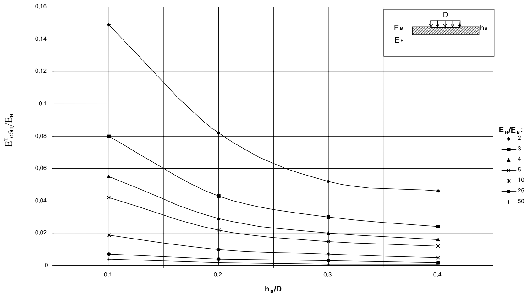
Рис. 2.7. Номограмма для расчета общего модуля двухслойной системы "теплоизолятор - подстилающий грунт". h_B - толщина слоя пенопласта; E_B - модуль упругости пенопласта; E_H - модуль упругости грунта.
